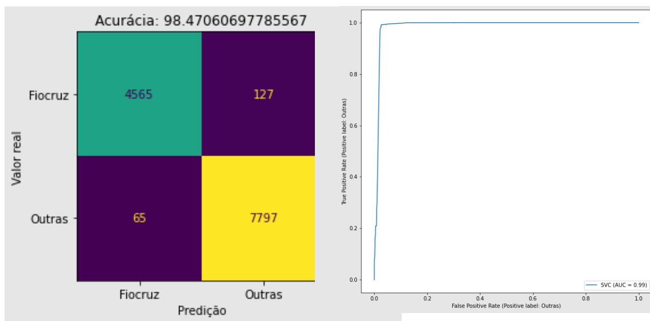
Figura 3: Curva ROC para o modelo de aprendizado de máquina.
